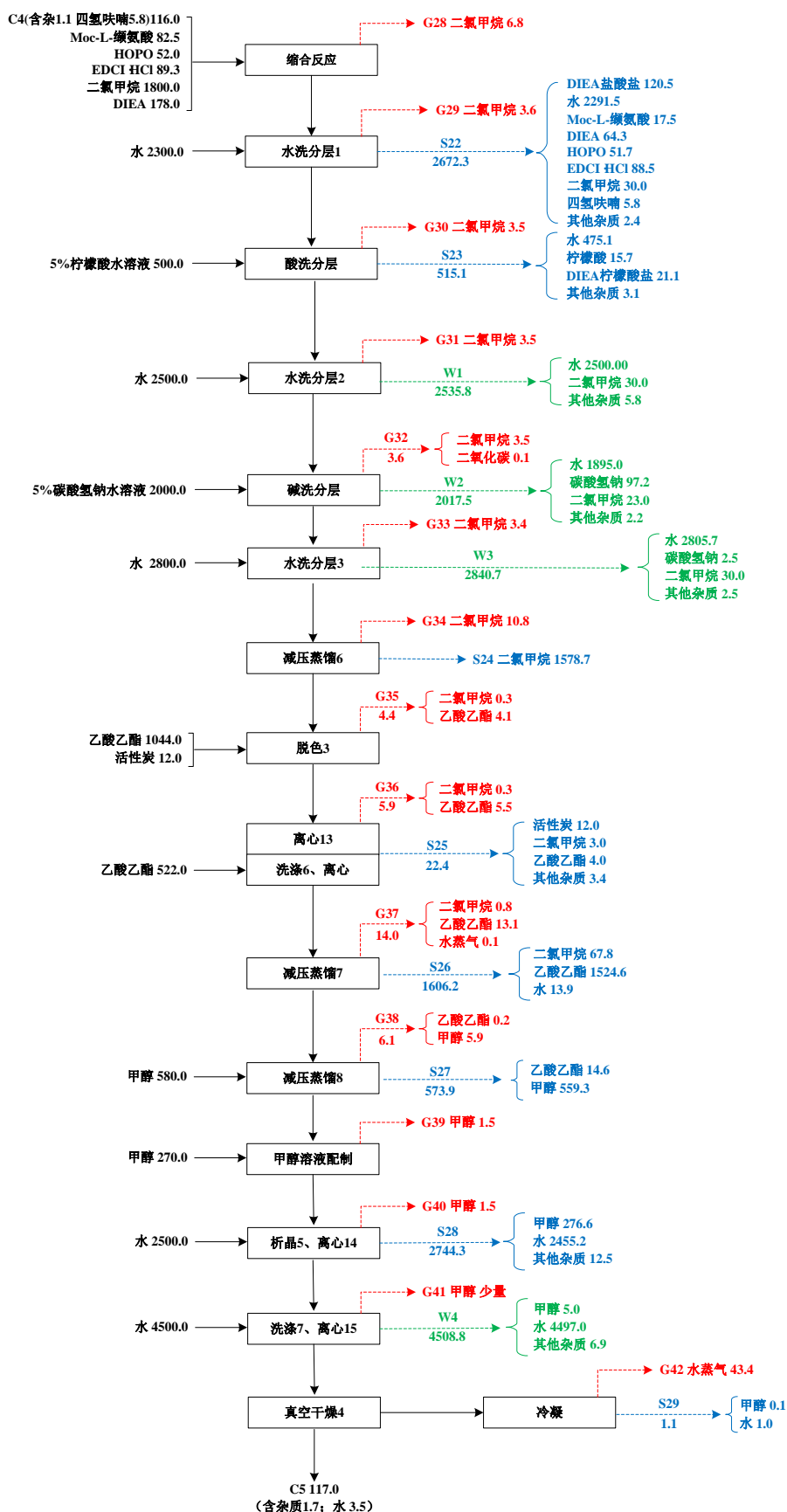
图 3.8-4 C5 中间体生产工艺流程及“三废”排放点位图（单位：kg/批）
