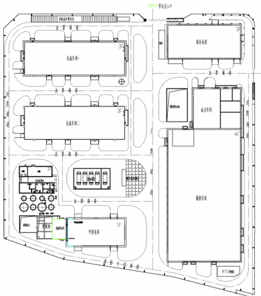
图 3.3-2 厂区平面布置图
