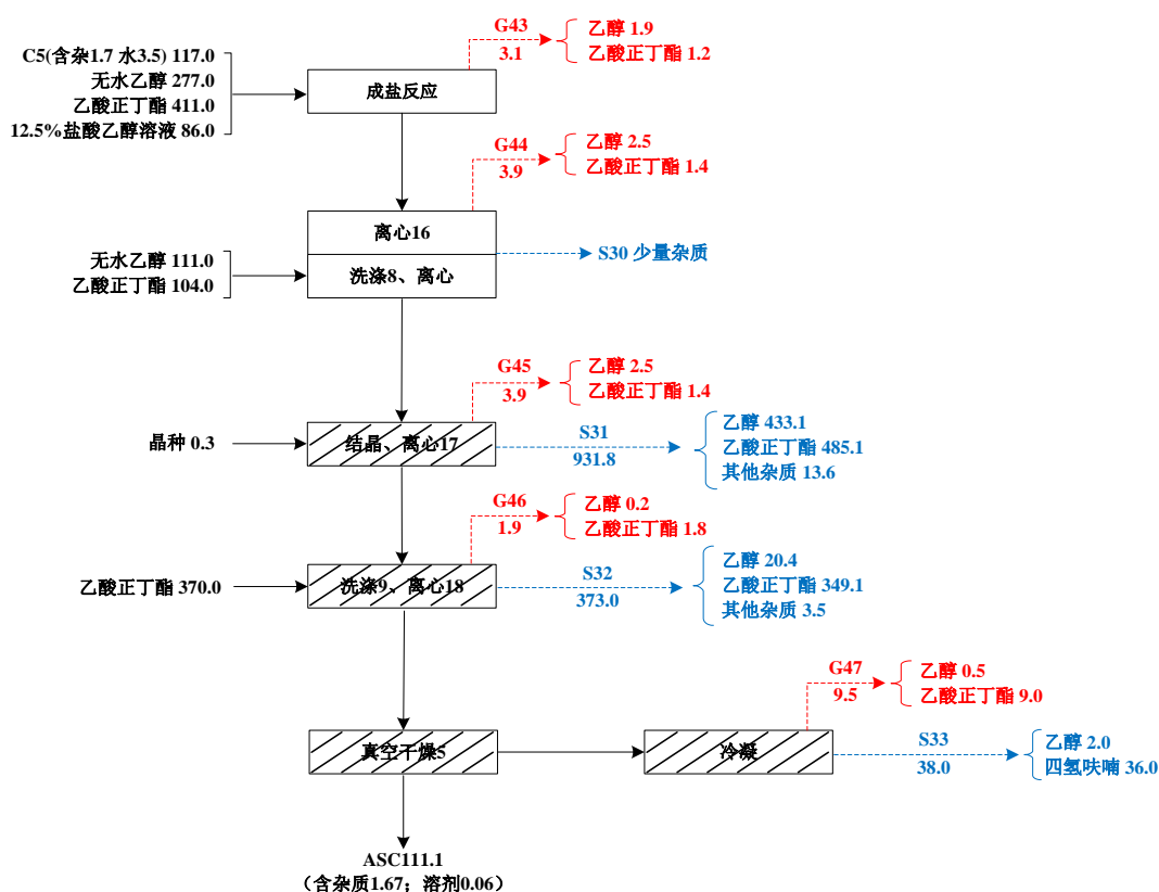
图 3.8-5 ASC16 成盐生产工艺流程及“三废”排放点位图（单位：kg/批）
