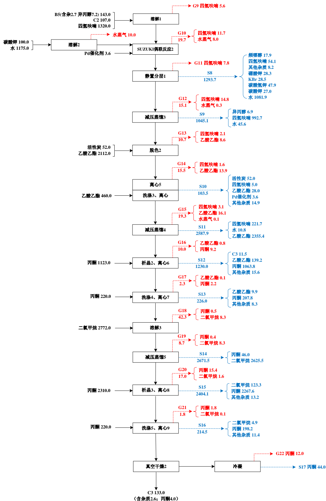
图 3.8-2 C3 中间体生产工艺流程及“三废”排放点位图（单位：kg/批）
