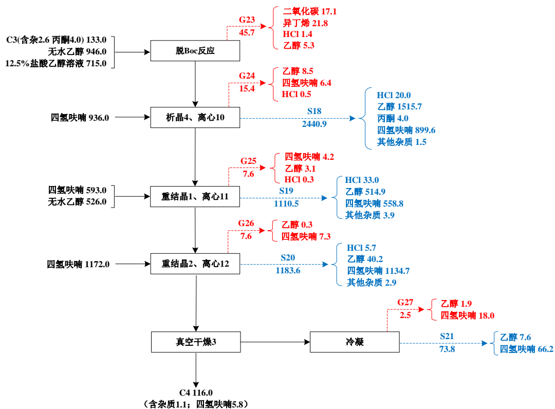
图 3.8-3 C4 中间体生产工艺流程及“三废”排放点位图（单位：kg/批）
