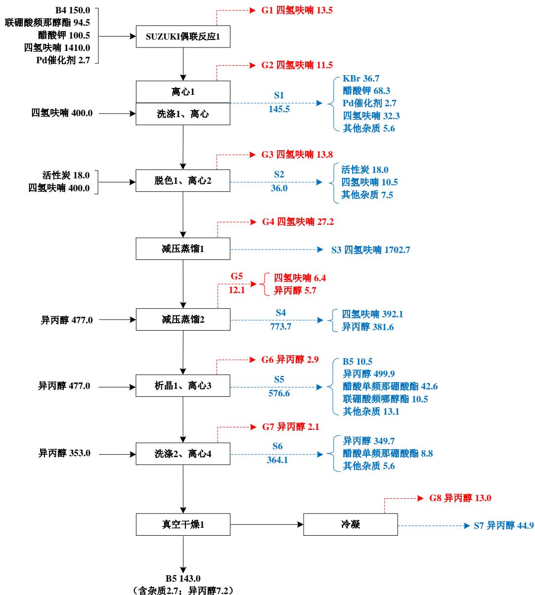
图 3.8-1 B5 中间体生产工艺流程及“三废”排放点位图（单位：kg/批）
